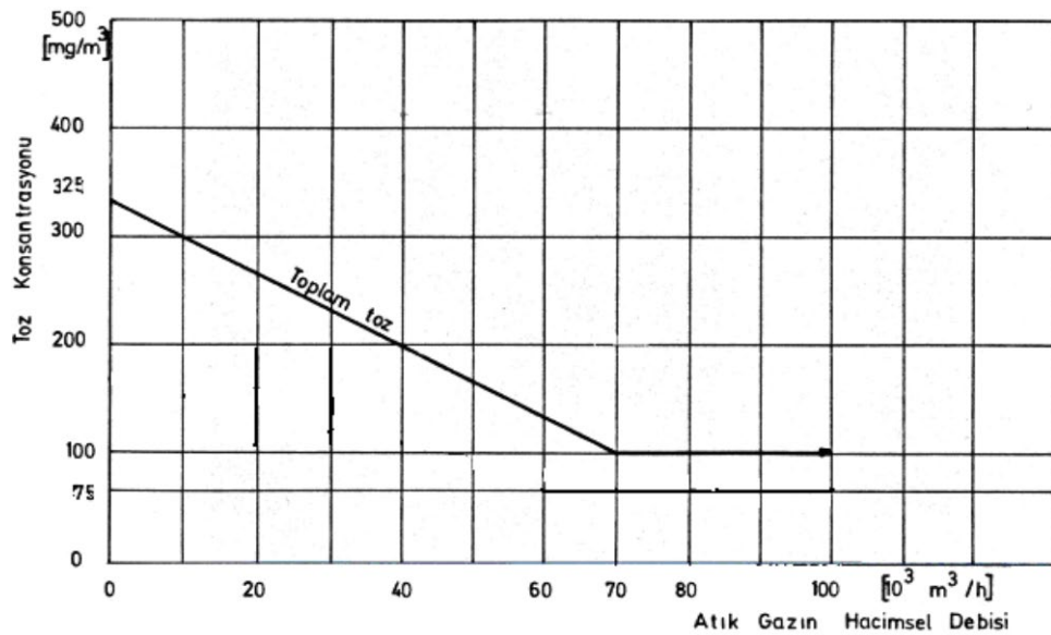
Diyagram 1 Toz Emisyon Sınırları
