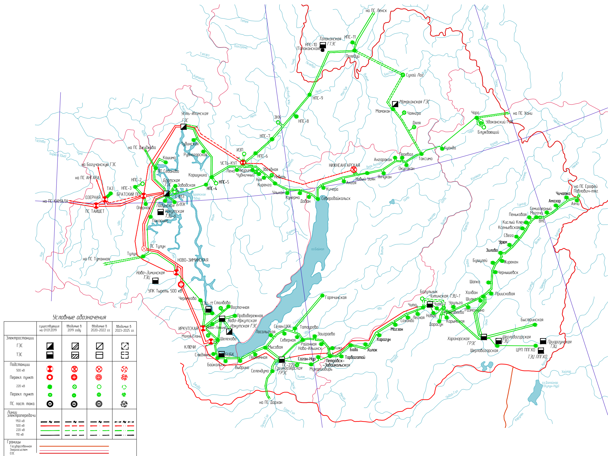
Карта-схема размещения линий электропередачи, подстанций напряжением 220 кВ и выше и электростанций Восточной Сибири на 2019–2025 годы
