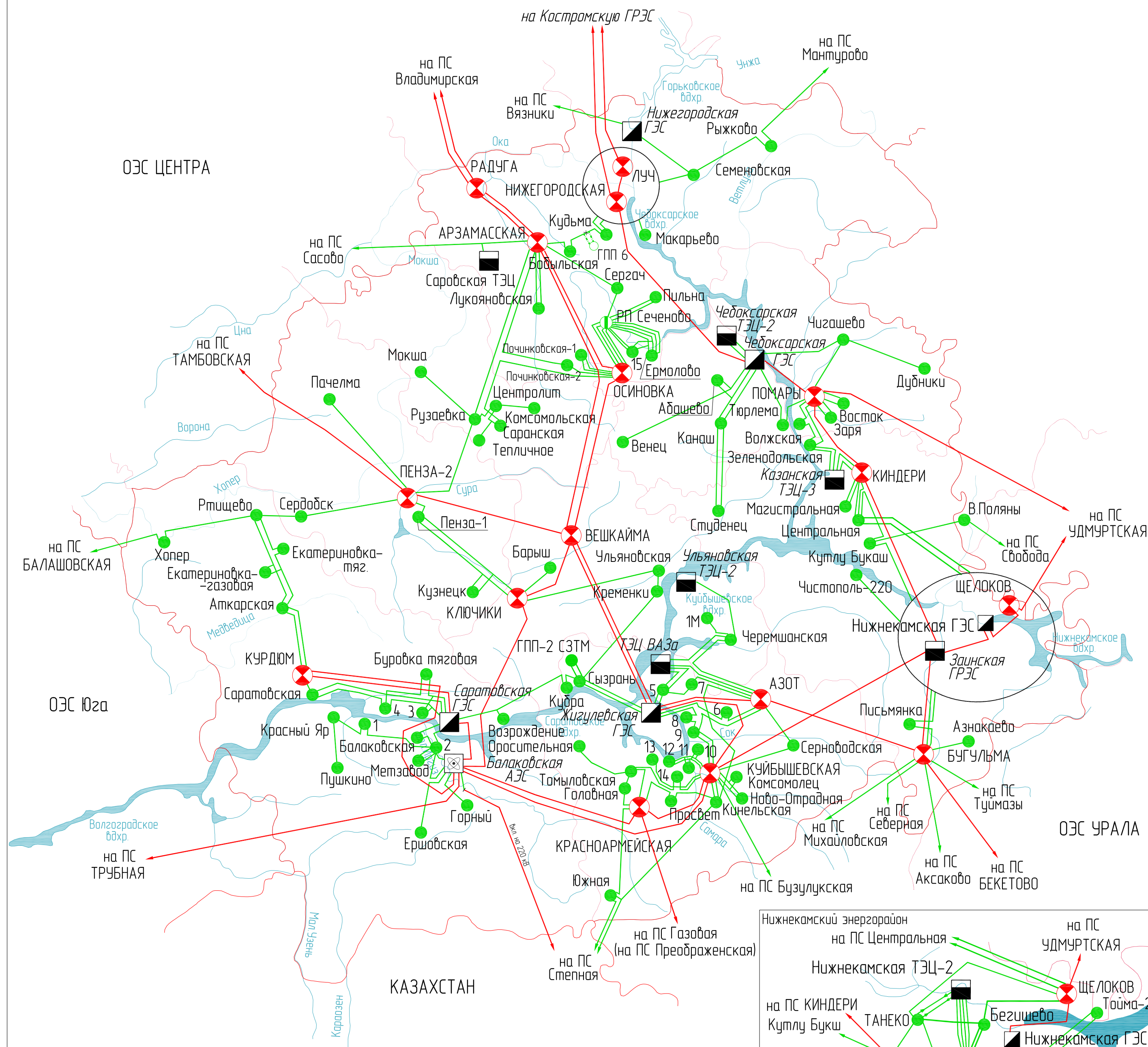
Карта-схема размещения линий электропередачи, подстанций напряжением 220 кВ и выше и электростанций ОЭС Средней Волги на 2019-2025 годы
