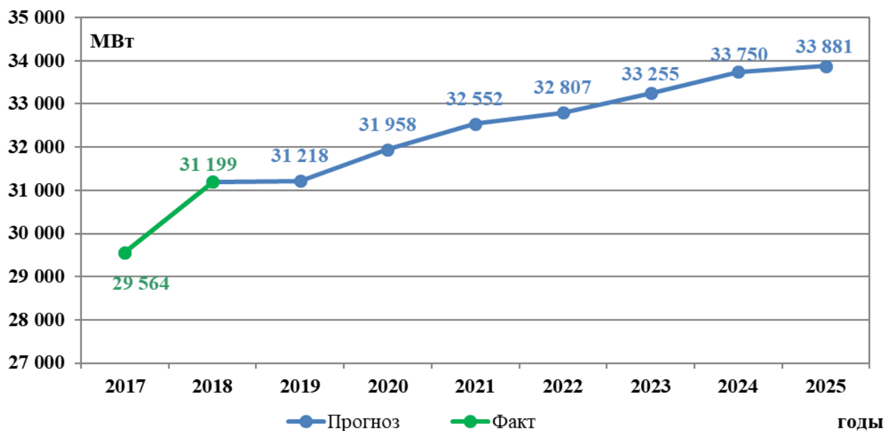
Рисунок 3.7 – Прогнозные значения собственного максимума потребления мощности ОЭС Сибири
