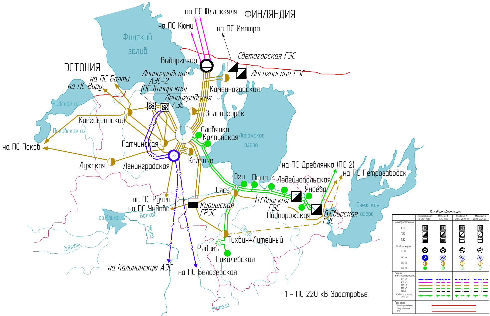
Карта-схема размещения линий электропередачи, подстанций напряжением 220 кВ и выше и электростанций Ленинградской энергосистемы на 2019-2025 годы
