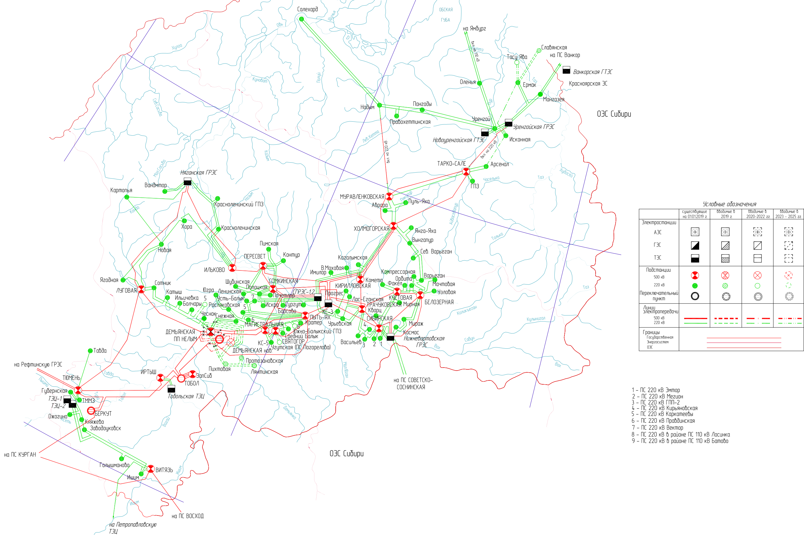
Карта-схема размещения линий электропередачи, подстанций напряжением 220 кВ и выше и электростанций энергосистемы Тюменской области на 2019–2025 годы
