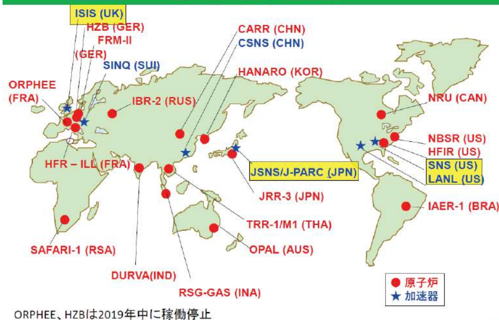
図 7-4 世界の中性子源
