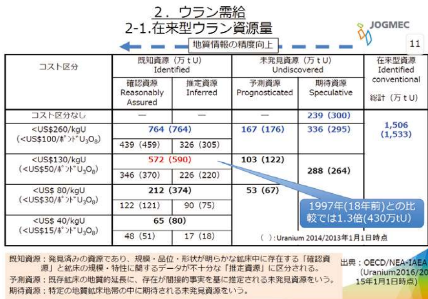
図 2-22 在来型ウラン資源量
