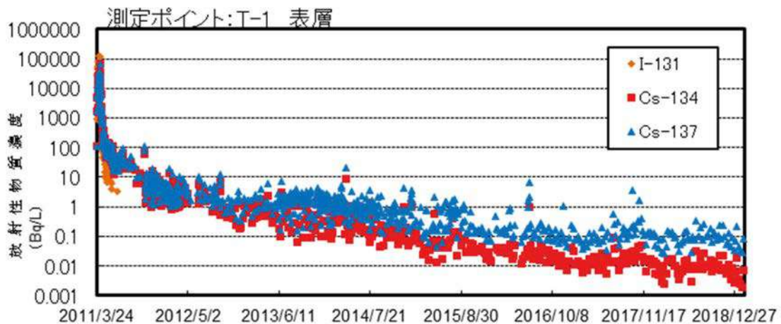
図 6-3 5、6号機放水口北側付近における放射性物質濃度の推移
