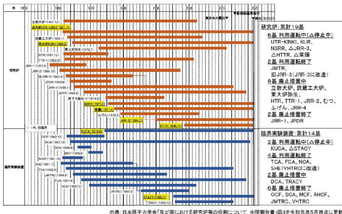
図 8-2 我が国の主な研究炉等施設
